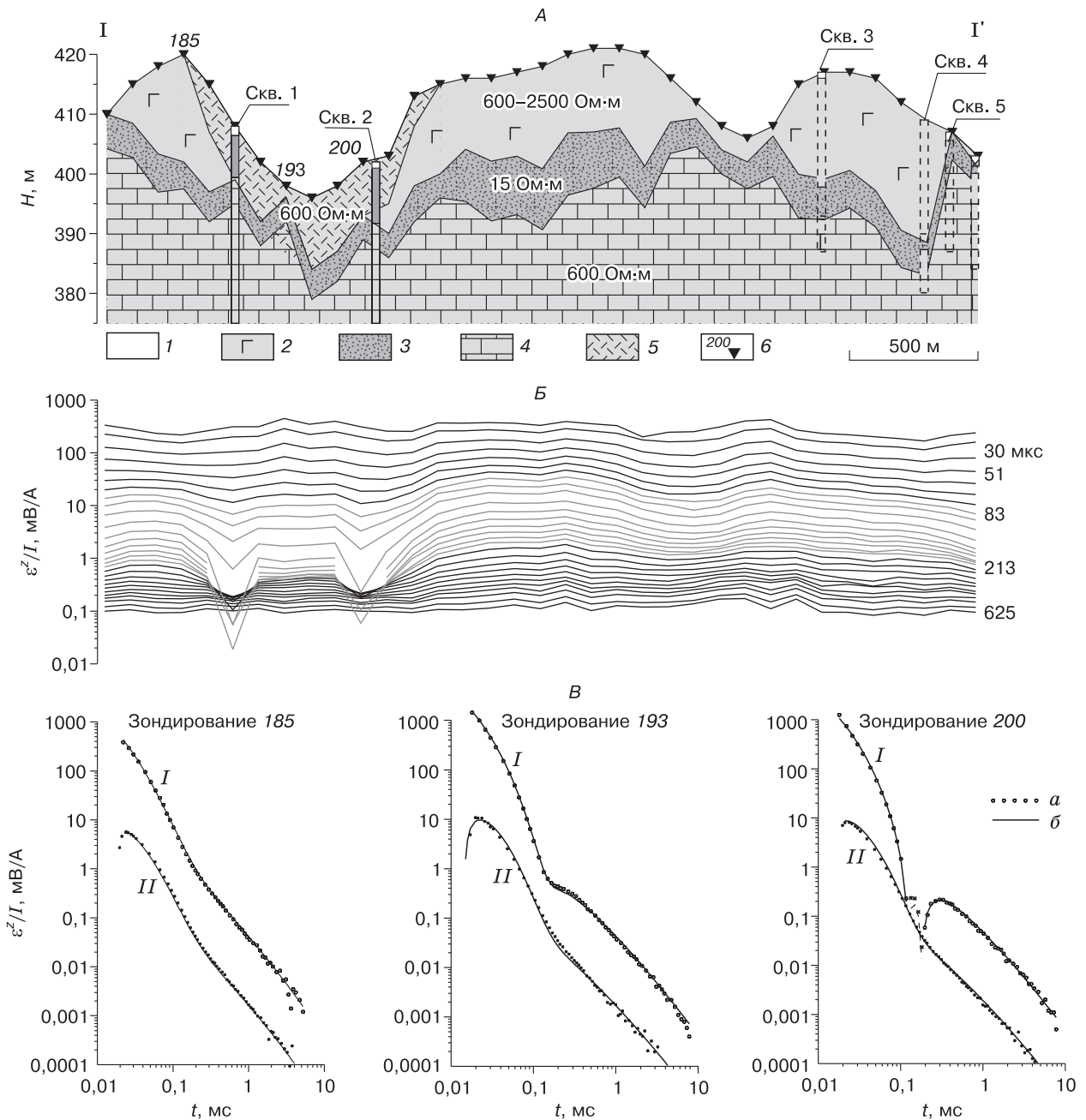
Рис. 5. Геолого-геофизический разрез по линии I–I', построенный по результатам одномерной инверсии с учетом поляризуемости среды (A), графики ЭДС по материалам измерения с совмещенной установкой 100 \times 100 м (B), измеренные и подобранные при инверсии кривые переходных процессов Верхне-Чуоналырского участка (B).
