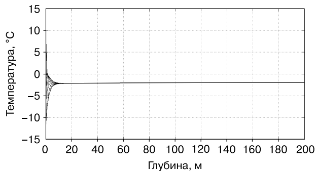
Рис. 2. Распределение температуры в массиве грунта в отсутствие сооружения:
