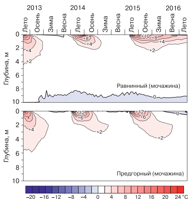
Рис. 3. Динамика температуры за 2013–2016 гг. в почвогрунтах мочажин.
