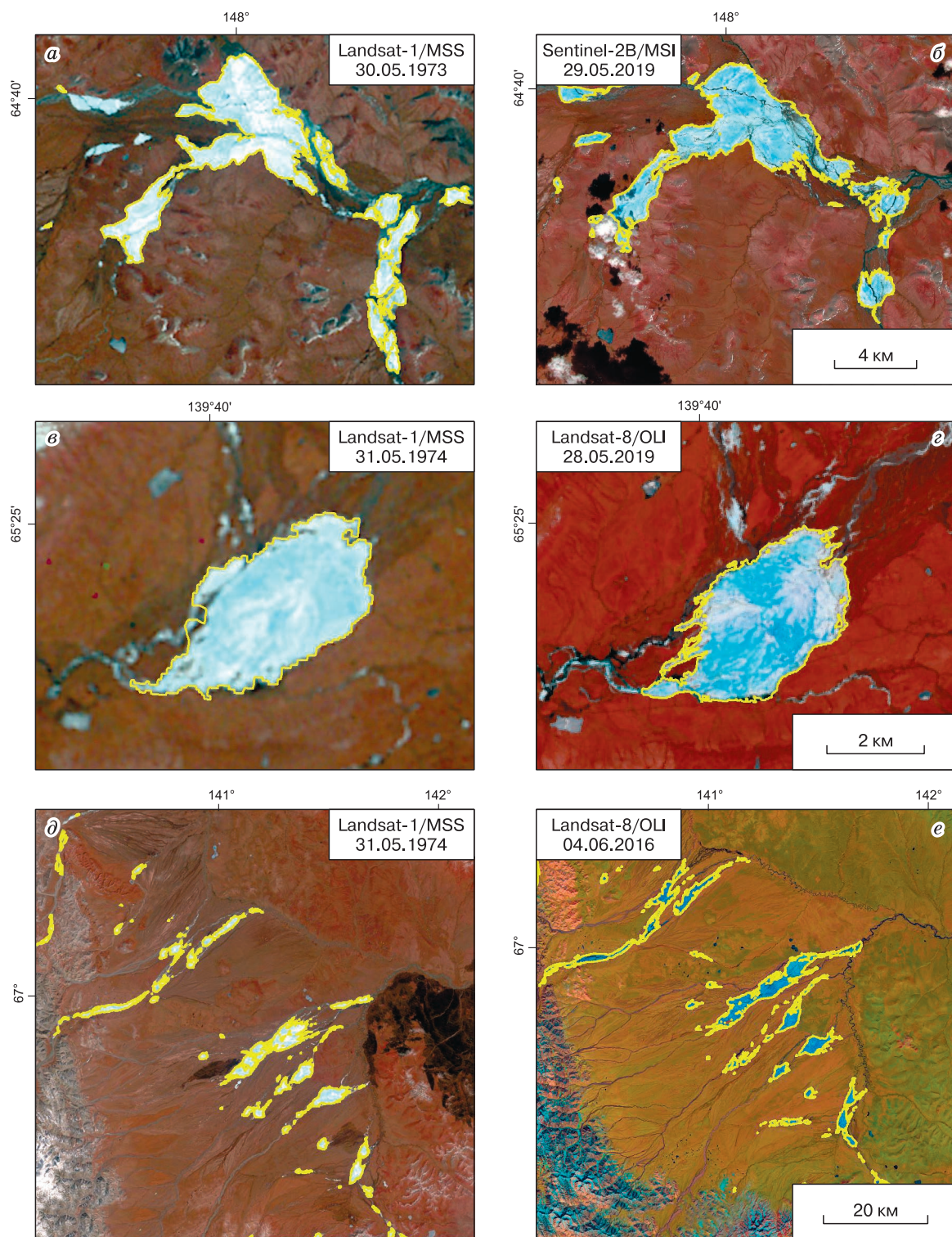
Рис. 5. Изменение площади отдельных гигантских наледей в бассейнах рек Колыма (а, б), Яна (в, з) и Индигирка (д, е) между 1973, 1974 и 2016, 2019 гг. по снимкам Landsat и Sentinel-2.
