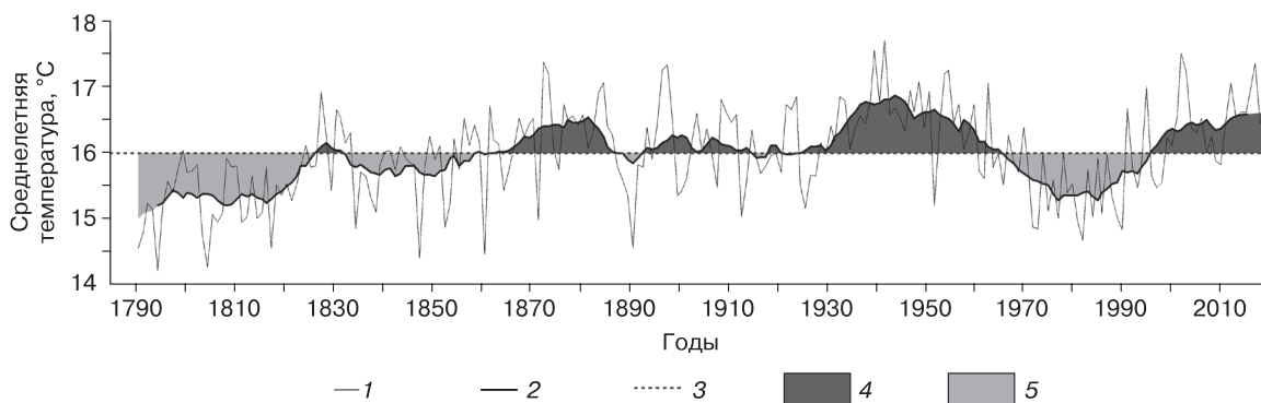
Рис. 4. Дендроклиматическая реконструкция летней температуры воздуха в районе Верхнеангарского хребта за последние 230 лет.
