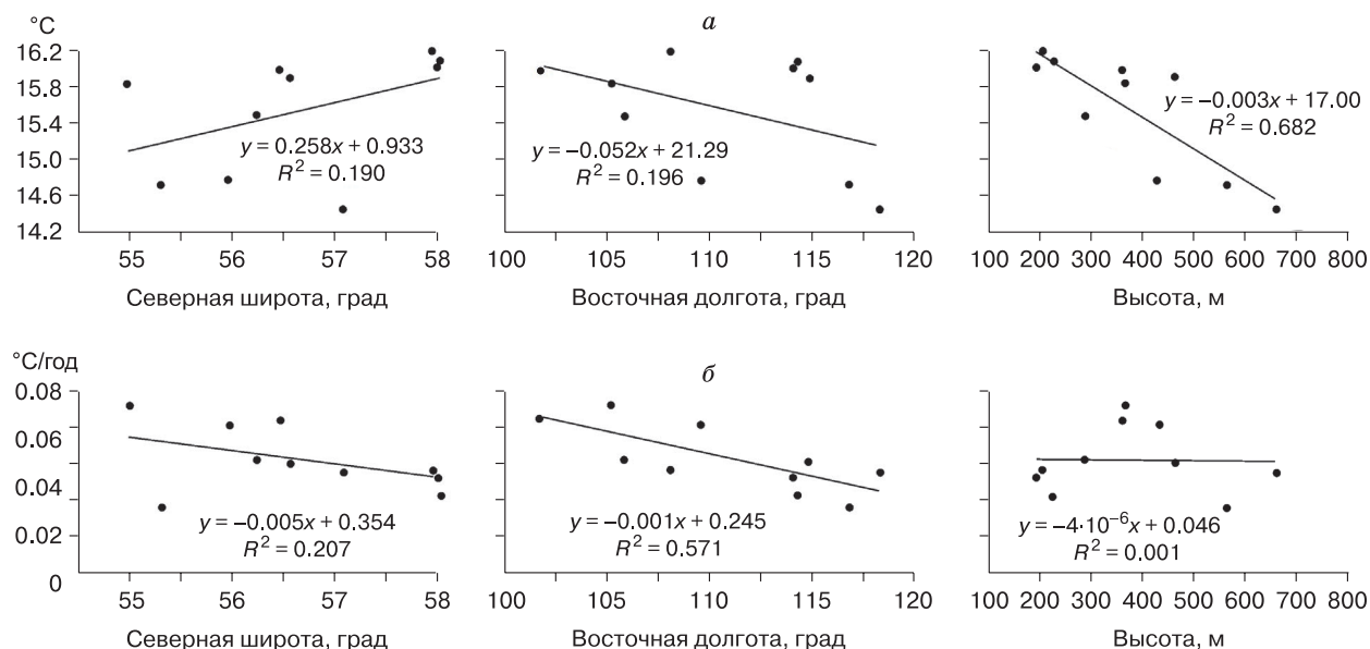
Рис. 3. Зависимость величины (а) и скорости повышения (б) средних летних температур от местоположения метеостанции.
