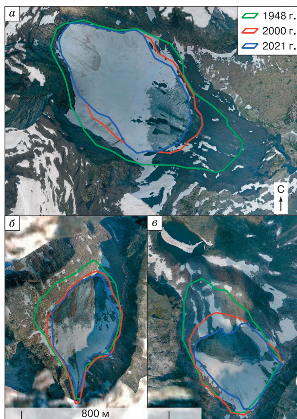
Рис. 5. Контуры ледников Черского (а), Урел-Амутис (б) и Огдында-Маскит (в) в 1948 г. (по данным аэрофотосъемки) и в 2000, 2021 гг. (по снимкам Landsat/Sentinel-2).
