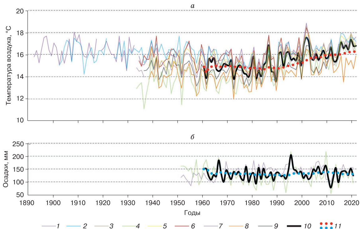
Рис. 2. Средняя летняя температура воздуха (а), определяющая абляцию, и осадки холодного периода, влияющие на аккумуляцию (б), по данным метеостанций:
