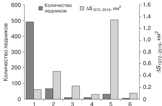
Рис. 8. Сокращение площади для ледников различных морфологических типов (определенных по Каталогу ледников СССР).
