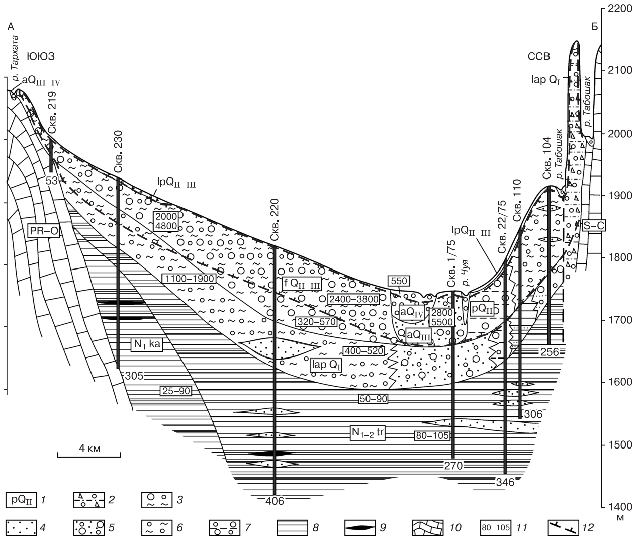
Рис. 2. Инженерно-геокриологический разрез по линии АБ по данным Чуйской партии гидрогеологической экспедиции 15-го района (1977 г.).
