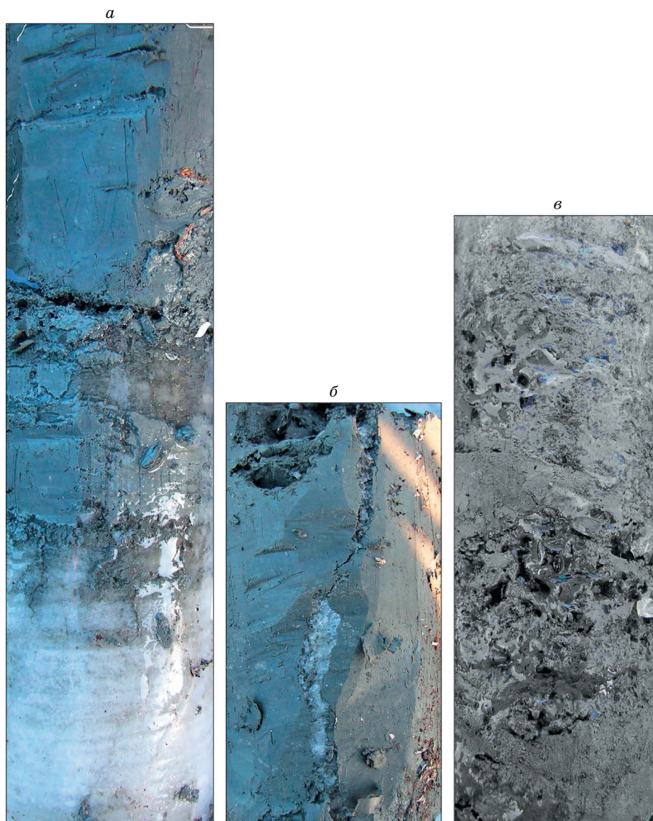
Рис. 3. Криогенная текстура суглинки, слагающего бугор на III озерно-аллювиальной равнине (а, б) и в тыловой части поймы р. Хейгияха (в).
