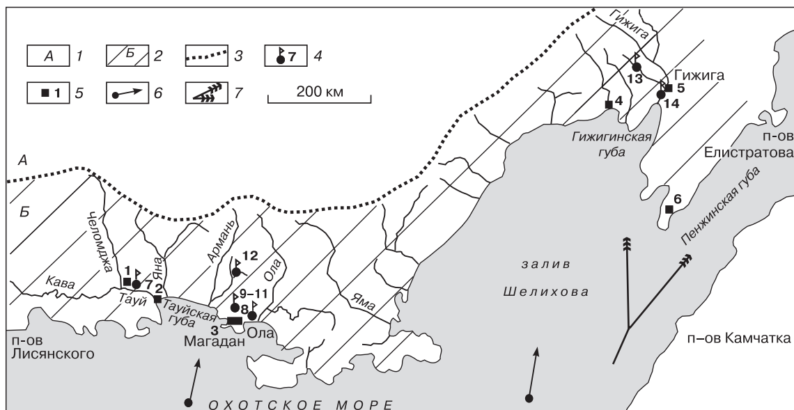
Рис. 1. Схематическая карта водосбора Примагаданского шельфа:
