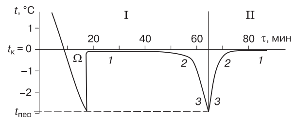
Рис. 1. Кривая замерзания (I) и оттаивания (II) песка.
