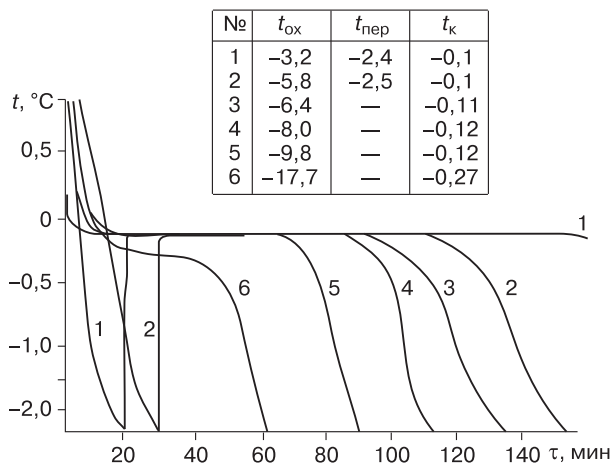
Рис. 2. Термограммы промерзающего грунта при разных значениях t_{\text{ох}} , t_{\text{пер}} и t_{\text{к}} в опытах 1–6.
