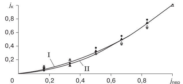
Рис. 7. Зависимость между величинами j_k и j_{\text{пер}} .
