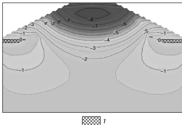
Рис. 1. Распределение температуры в основании насыпи высотой 6 м в конце периода охлаждения 50-го года эксплуатации.
