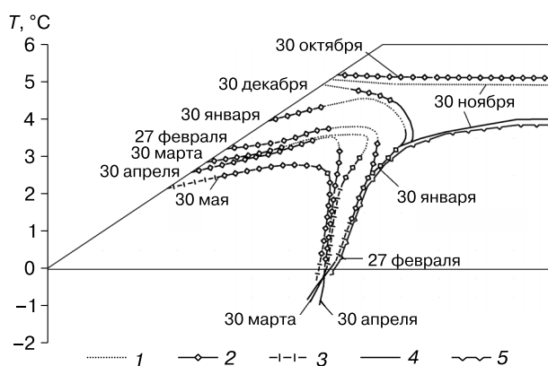
Рис. 4. Величина градиентов температуры грунтов у фронта промерзания по результатам моделирования температурного поля:
