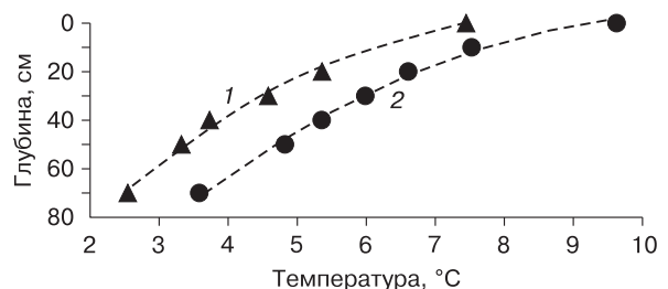
Рис. 4. Распределение по глубине средней температуры породы за период 06.07–08.08.2016 г. под мхом толщиной 5 см (1) и 1 см (2).
