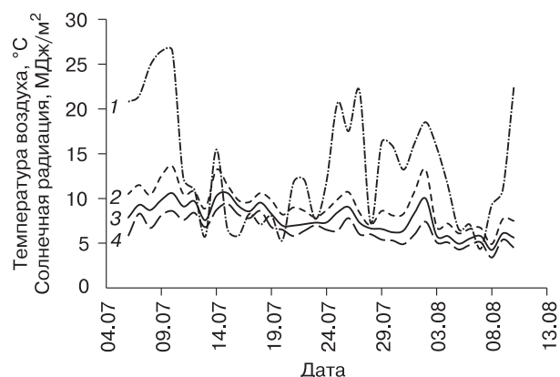
Рис. 1. Динамика суммарной солнечной радиации (1) и температуры воздуха.
