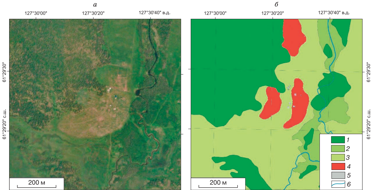
Рис. 7. Космоснимок местности Амчях (а) и результаты его дешифрирования (б).
