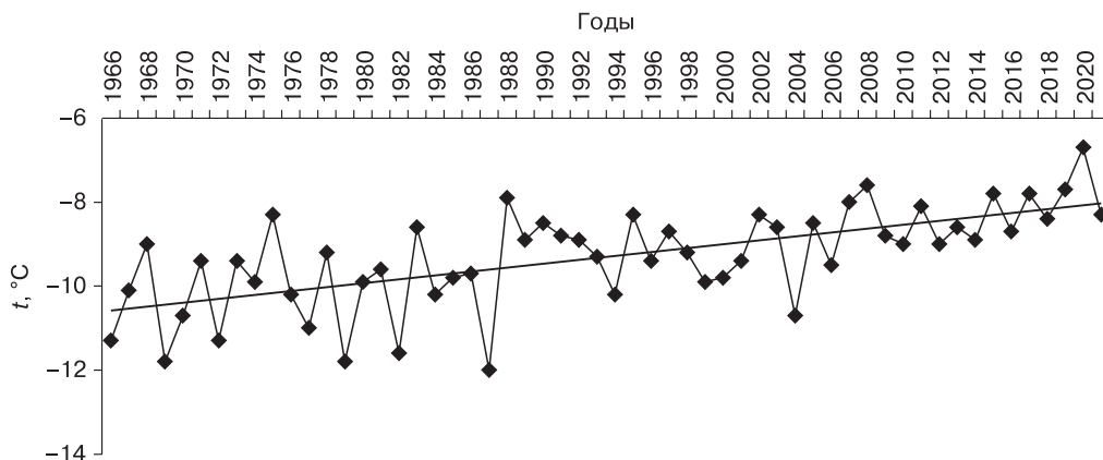
Рис. 3. Динамика среднегодовой температуры воздуха t в 1966–2021 гг. по данным Покровской метеостанции.
